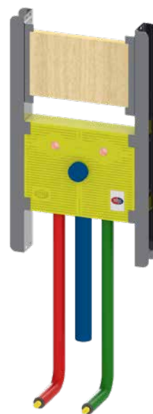
Figur 3B6 – Set Waschtischbox und Traverse
