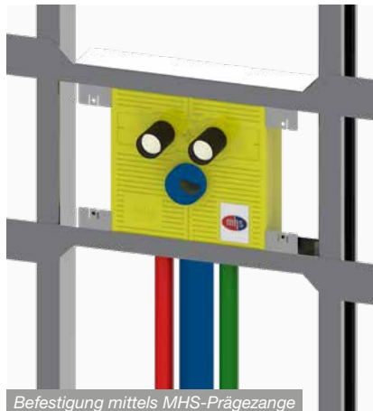
Befestigung mittels MHS-Prägezange
