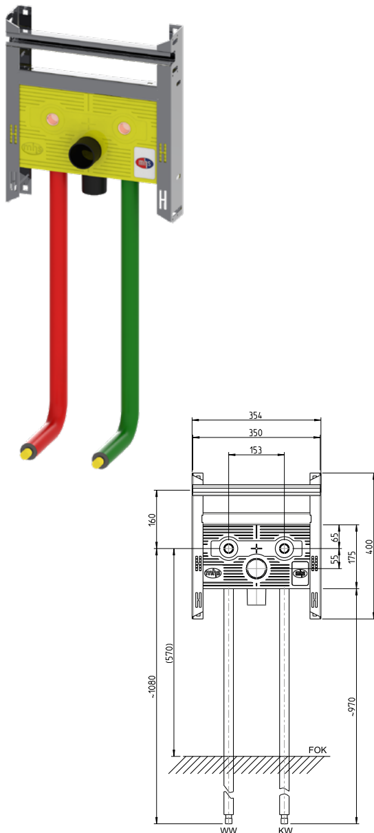
Figur 314 – Set Waschtischbox und Traverse
