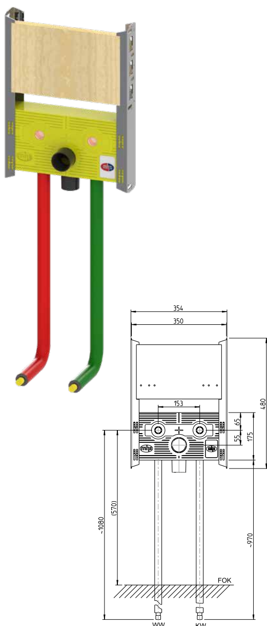
Figur 315 – Set Waschtischbox und Traverse
